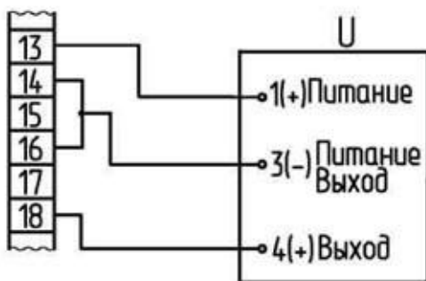
Рисунок В.5 - Схема с BSPТ-10M Остальное - см. рисунки В.1 или В.2
